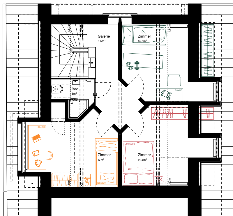
Grundriss Dachgeschoss
