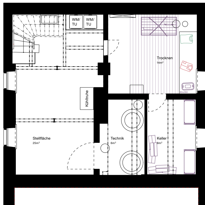
Grundriss Untergeschoss
