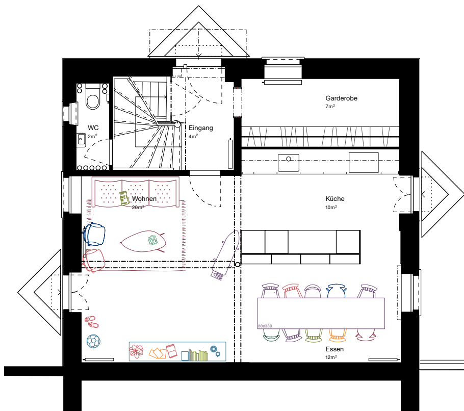
Grundriss Erdgeschoss
