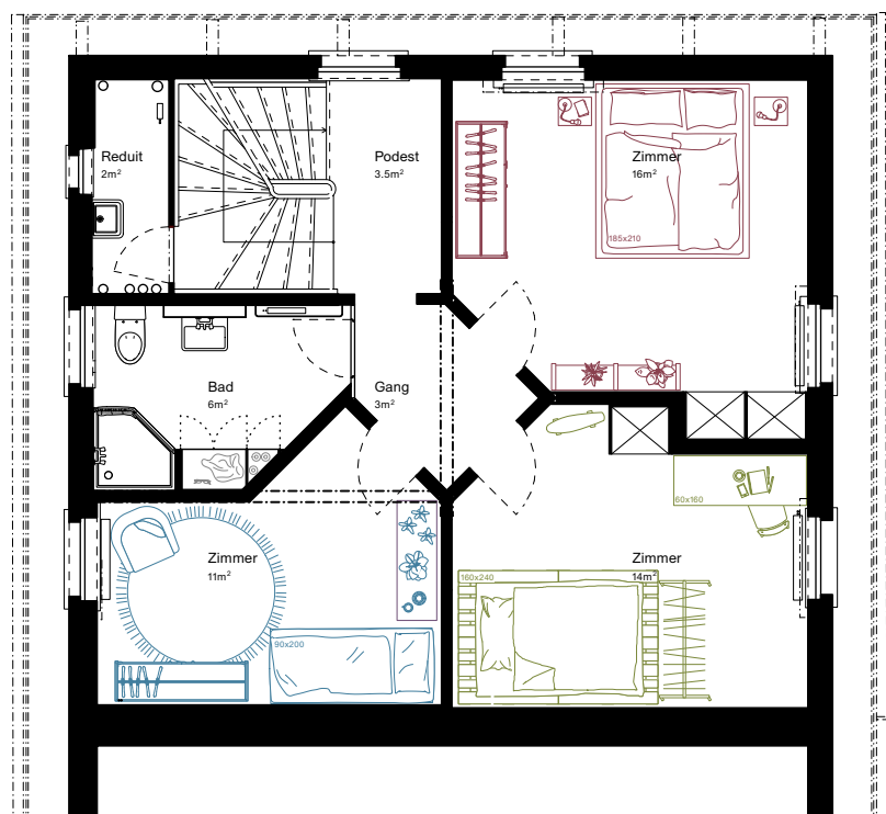
Grundriss 2. Obergeschoss
