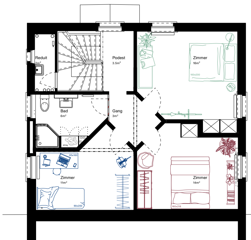
Grundriss 1. Obergeschoss
